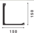
L1 ARSTYL® 150 x 150 x 2000mm
